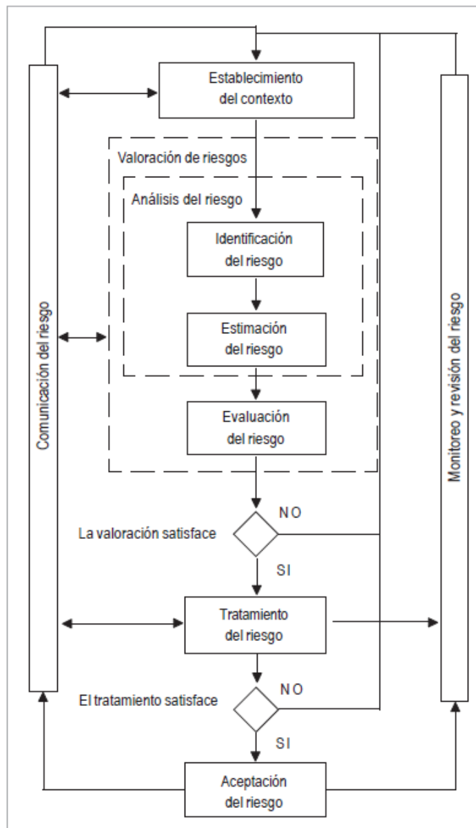
Imagen 4. Proceso para gestión de riesgos de acuerdo con ISO 27005
